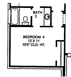
OPTIONAL BEDROOM #4 IN LIEU OF STUDY
